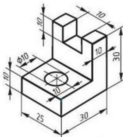
Рисунок 1 - Пример изделия
